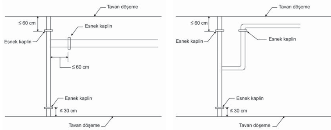
Şekil 9.5.2.3 Çok Katlı Binalarda Esnek Kaplin Yerleşimi
