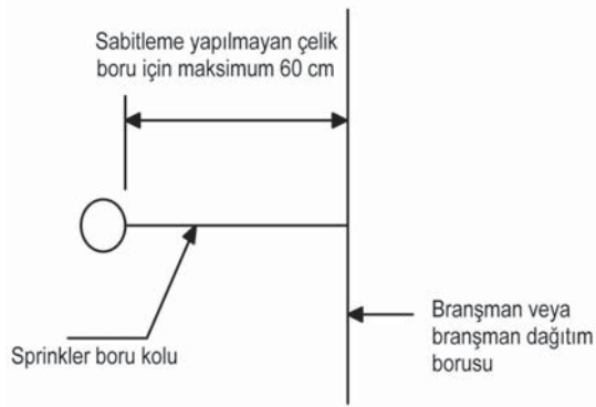
Şekil 9.4.1.6(a) Sabitleme Yapılmayan Boru Kolu Mesafesi
