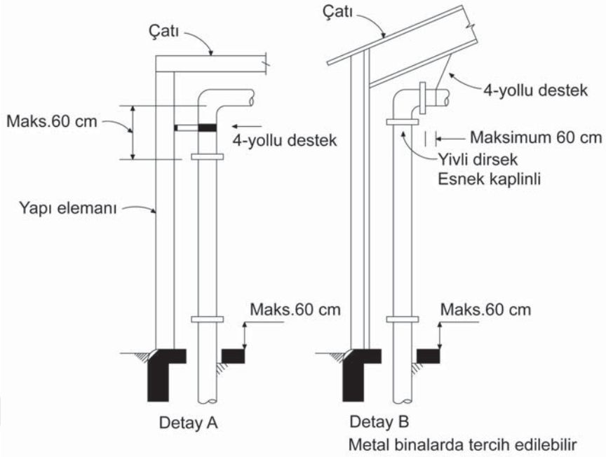
Şekil 9.5.5.1(a) 4-yollu Destek Yerleşimi
