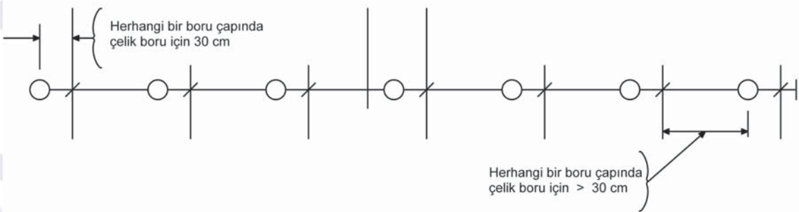
Şekil 9.4.1.5(b) En Son Sprinklerin Boru Askılarına Mesafesi
